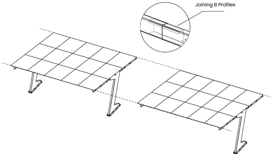
Fig. 28. Extension of the Carport Avrii SOL Integra Zcon
